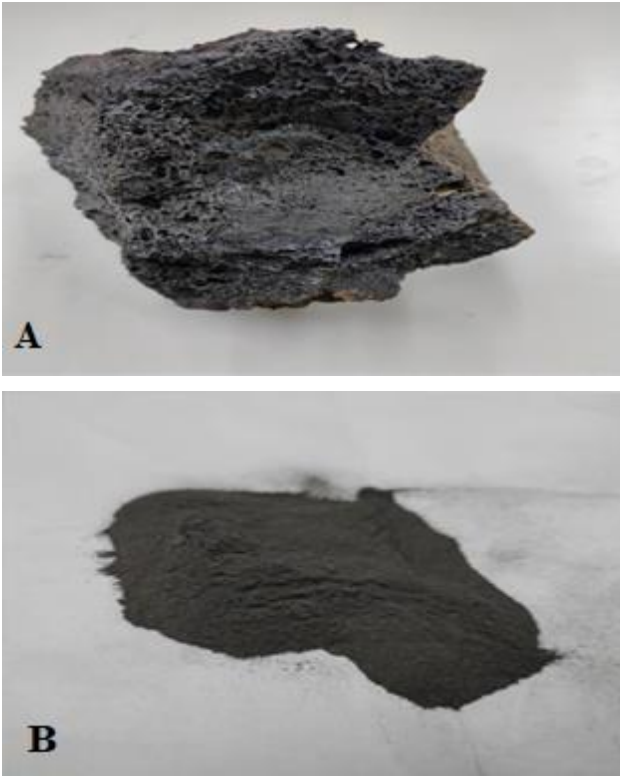
Şekil 1. (A) BR1'in kayaç hali. (B) BR1'in (-80, +100 mesh) tanecikli boyutlu hali.
